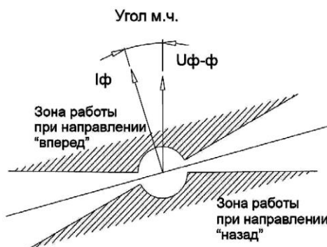
Рис. 6. Работа направленной защиты от замыканий на землю
