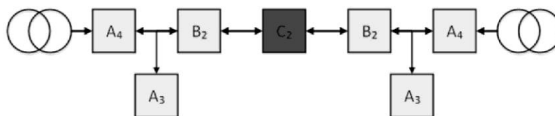
Рис. 4. Сеть с двусторонним питанием
