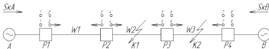
Рис. 5. Работа направленной защиты максимального тока.
